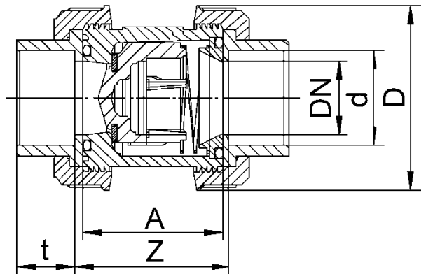
Rückschlagventil S6
