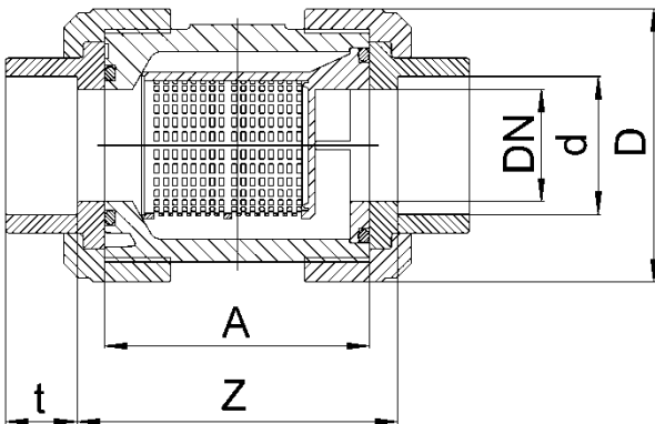
Schmutzfilter S4
