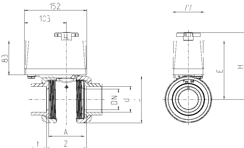
PVC Kugelhahn DN32 – DN50 S6 E0510 ECO 230V
